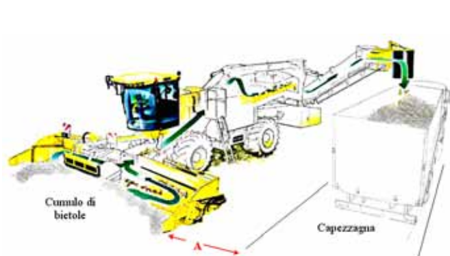
Figura 1. Posizione del cumulo tale da consentire la piena operatività della macchina sterratrice. Le macchine più grandi necessitano di circa 6 m di spazio.
