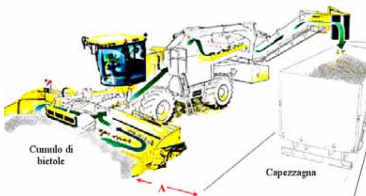
Figura 1. Posizione del cumulo tale da consentire la piena operatività della macchina sterratrice. Le macchine più grandi necessitano di circa 6 m di spazio.
